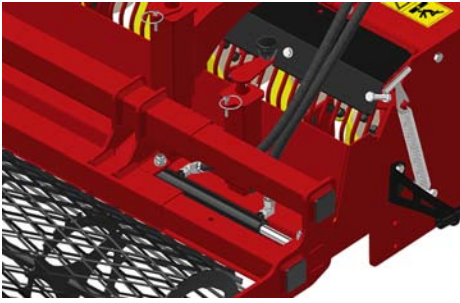
Option : Déplacement hydraulique du châssis rouleau métal déployé
