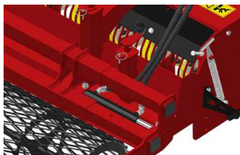
Option : Déplacement hydraulique du châssis rouleau métal déployé (de série avec rouleau en fonte)
