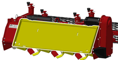
Système d'attache rapide conventionnel
